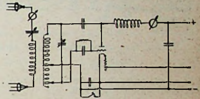
SCHEMA-öKE.
